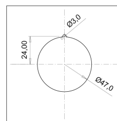
SOMUNLU PANO PRİZİ MONTAJ DELİĞİ ÖLÇÜLERİ
