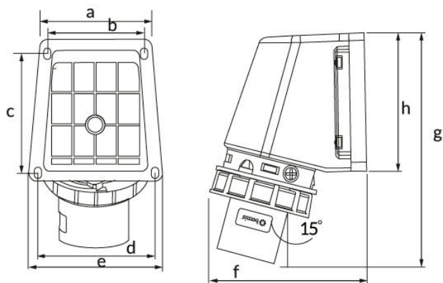
Ölçüler / Dimensions (mm)
