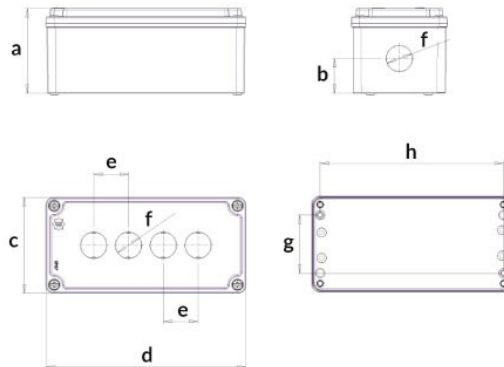
Ölçüler / Dimensions (mm)
