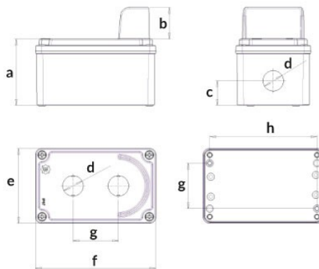
Ölçüler / Dimensions (mm)
