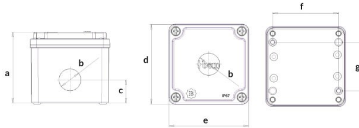
Ölçüler / Dimensions (mm)
